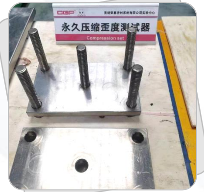
永久压缩变形实验
